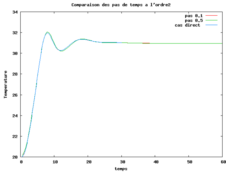
Figure 4.11: FreeFem++ : Evolution thermique de X2 à différents pas de temps. Le cas direct correspond au cas où l'on passe directement à l'ordre 2 (cf. 2.2.4).
