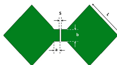
Fig. 1. Diamond Dipole.
