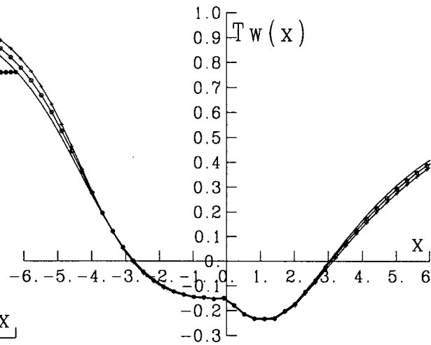
Fig. 2. - Frottement pariétal.
