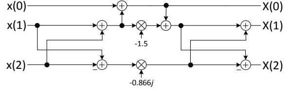
(b) Radix-3
