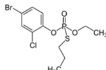
Profenofos log P = 4.68
