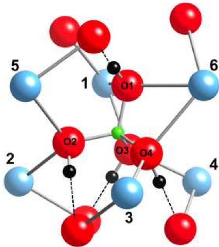
calcite
