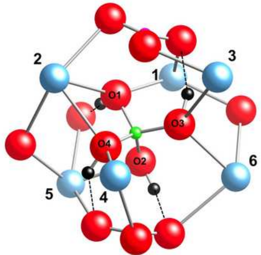
aragonite
