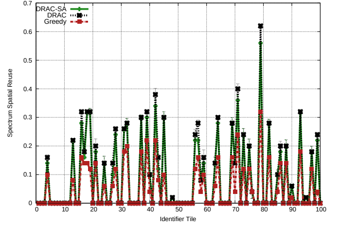
Fig. 5: SSR per PRB, SINR = 25 dB
