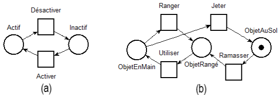
Figure 3 • Modélisation d'un objet activable (a) et d'un objet ramassable (b) à l'aide de mini-réseaux de Petri simples
