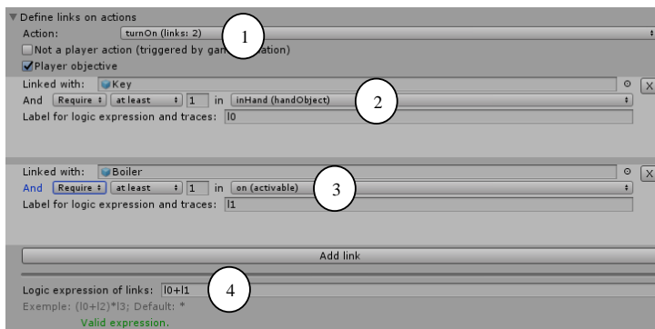
Figure 6 • Capture d'écran du module d'édition du suivi.
