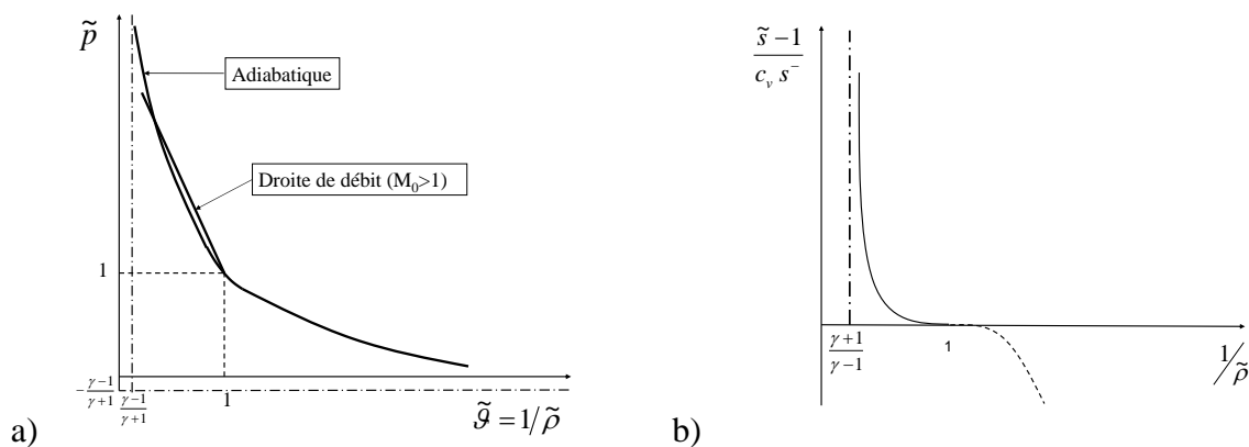
Figure 9. L'adiabatique d'Hugoniot dans les plans a) \tilde{g}, \tilde{p} et b) \tilde{s}, \tilde{s}^- . Le nombre de Mach de l'écoulement amont par rapport à l'onde est : M^- = M_0 = u_0/c_0 . Il n'y a de choc que pour M^- > 1 . La droite de débit a pour équation : (\tilde{p} - 1)/(\tilde{g} - 1) = -\gamma M_0^2 .
