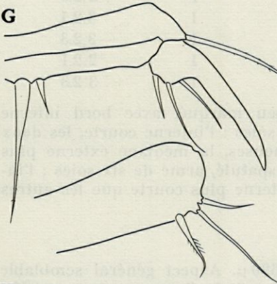
PLANCHE 3. — Stenhelia ( D. ) coineauae n. sp. Femelle : A, P1. B, P2. C, P3. D, P4. E, P5. Mâle : F, endopodite de P2. G, P5. H, P6.
