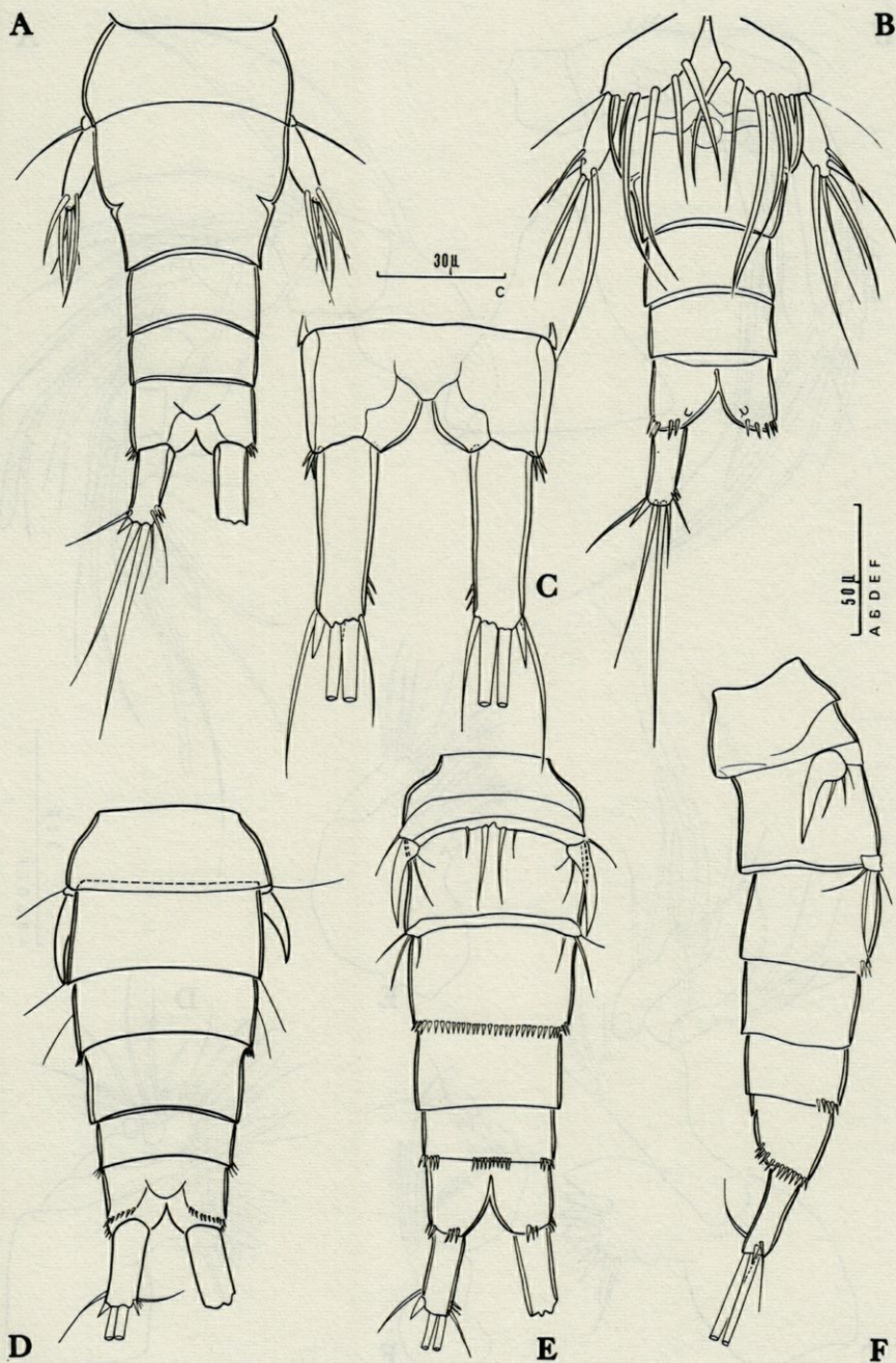
PLANCHE 1. — Stenhelia (D.) coineauae n. sp. Femelle : A, urosome (vue dorsale); B, urosome (vue ventrale); C, rames furcales. Mâle : D, urosome (vue dorsale); E, urosome (vue ventrale); F, urosome (vue latérale).
