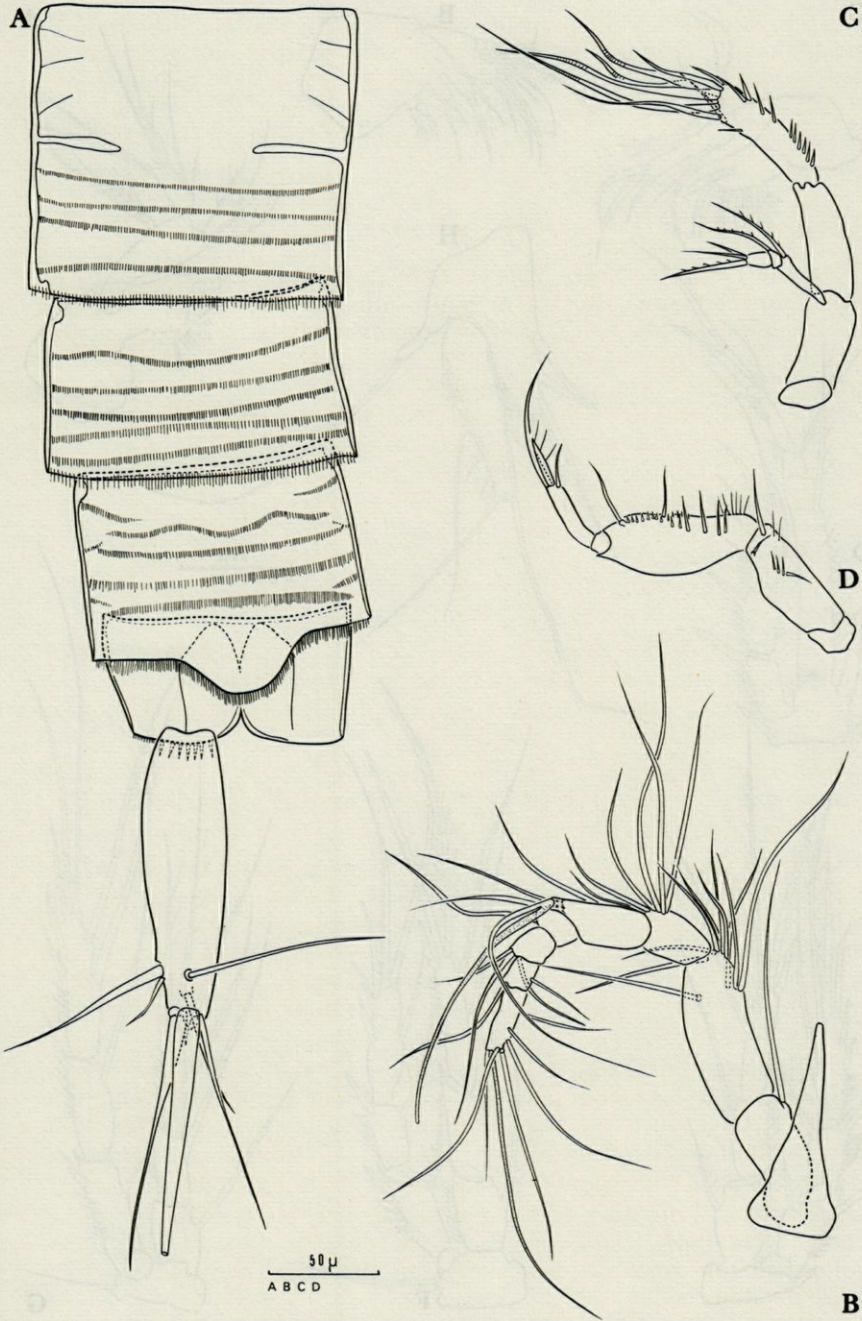
PLANCHE 6. — Typhlamphiascus bouligandi n. sp. Femelle : A, urosome et rame furcale (vue dorsale). B, antennule et rostre. C, antenne. D, maxillipède.
