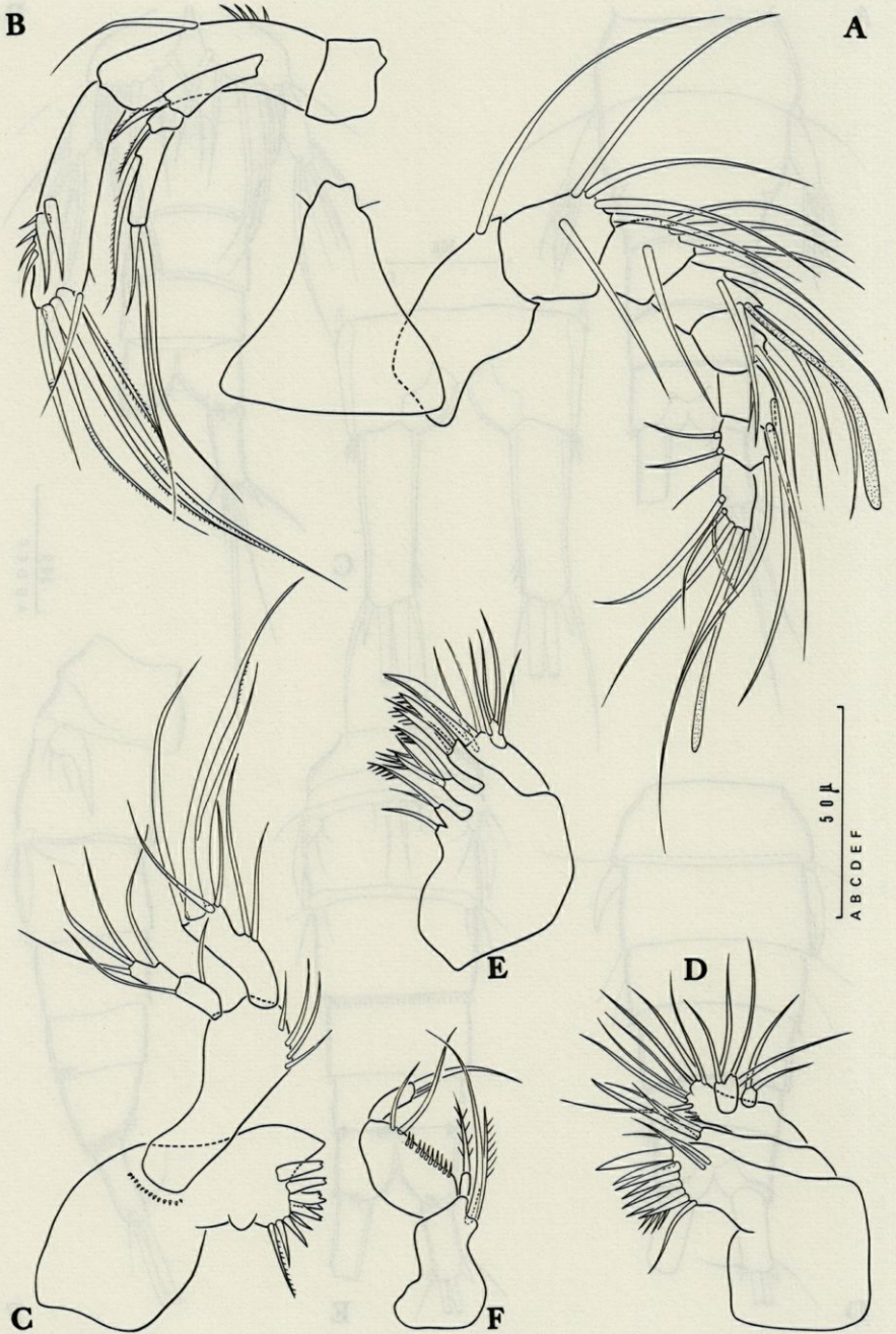
PLANCHE 2. — Stenhelia (D.) coineauae n. sp. Femelle : A, antennule et rostre. B, antenne. C, mandibule. D, maxillule. E, maxille. F, maxillipède.
