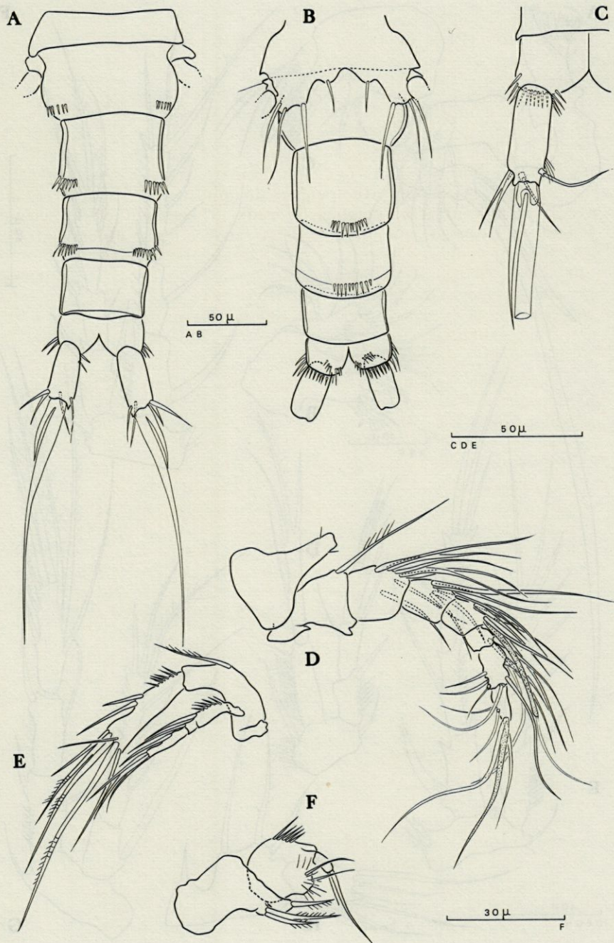
PLANCHE 4. — Stenhelia (D.) bocqueti n. sp. A, urosome (vue dorsale). B, urosome (vue ventrale). C, rame furcale. D, antennule et rostre. E, antenne. F, maxillipède.
