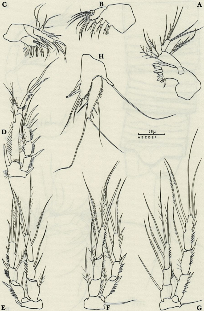
PLANCHE 7. — Typhlamphiascus bouligandi n. sp. Femelle : A, mandibule. C, maxillule. B, maxille. D, P1. E, P2. F, P3. G, P4. H, P5.
