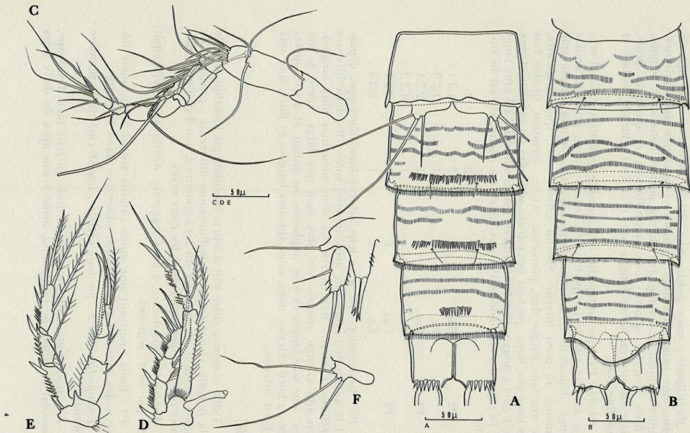
PLANCHE 8. — Typhlamphiascus bouligandi n. sp. Mâle : A, urosome (vue ventrale). B, urosome (vue dorsale). C, antennule. D, P1. E, P2. F, P5 et P6.
