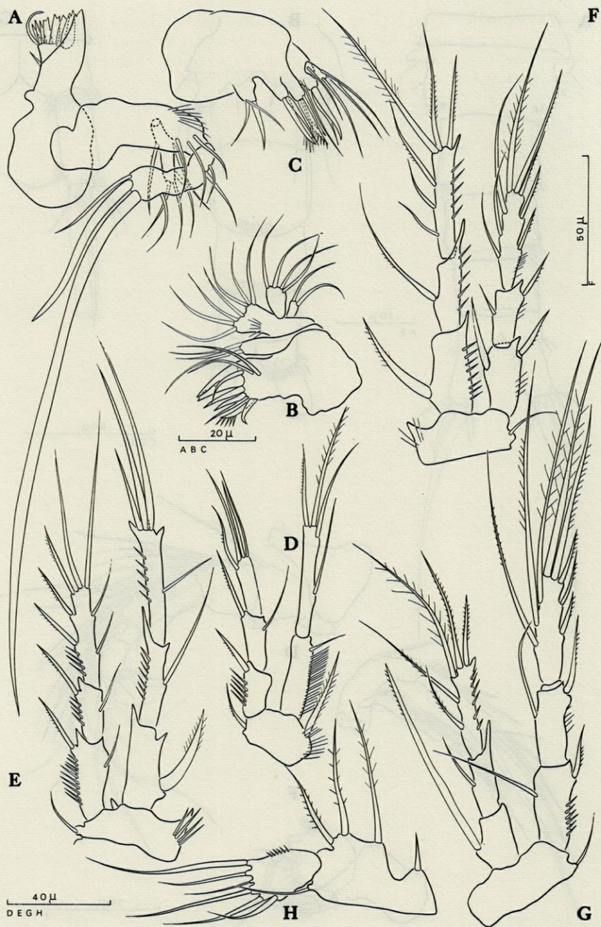
PLANCHE 5. — Stenelia (D.) bocqueti n.sp. A, mandibule. B, maxillule. C, maxille. D, P1. E, P2. F, P3. G, P4. H, P5.
