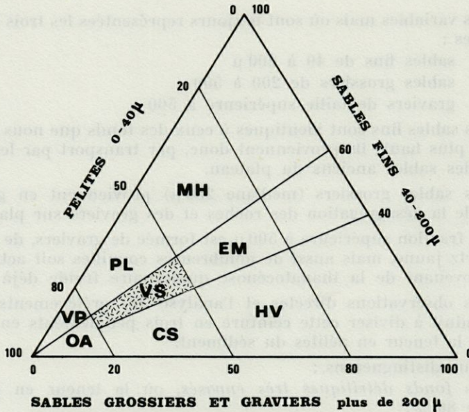
DIAGRAMME 5 : granulométrie du détritique envasé à Venus-Spatangus .
