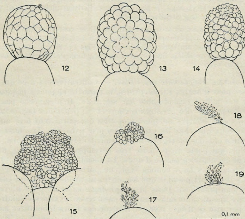
Figs 12 à 19. — Amallocystis boschmai . — Evolution des gonomères distaux. — 12. Stade à réseau polygonal superficiel. Remarquer aussi le funicule apical. — 13. Stade à demi-sphères. — 14. Stade à « perles » pédiculisées. Les boursouflures distales sont subdivisées. — 15. Subdivision plus avancée des « perles ». — 16. Rudiments de sporulation sur la partie apicale d'un gonomère distal. — 17 à 19. Derniers rudiments laissés par le gonomère distal sur l'extrémité apicale du gonomère suivant.
