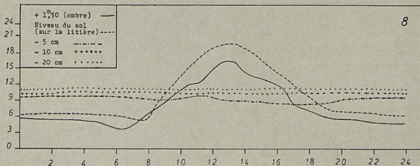
Fig. 8. — Variations journalières de température d'un sol brun forestier. Versant sud des Pyrénées occidentales, forêt de hêtres, avec litière de 7 à 8 cm, alt. 900 m, au voisinage de la station 13. Août, journée ensoleillée avec quelques passages de nuages surtout l'après-midi. L'évaporation consécutive à une pluie de la veille détermine un abaissement diurne de la température dans les couches superficielles du sol.
