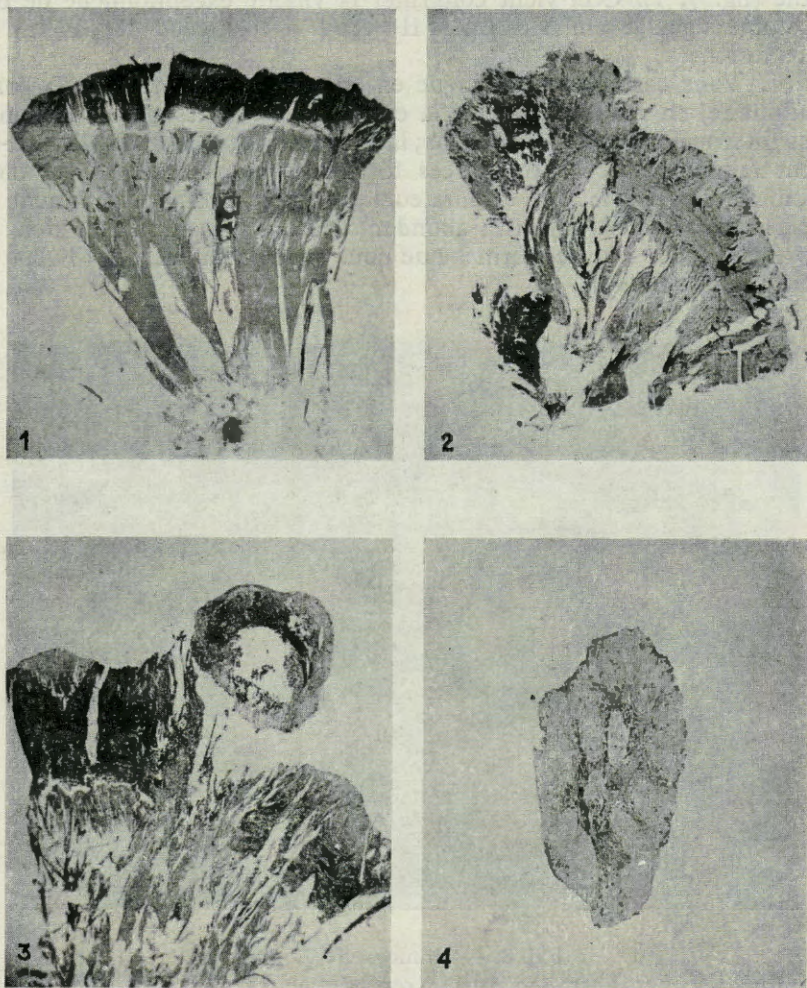
Fig. 7. — Homogreffe Tethya
