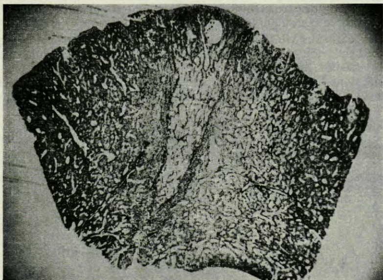
Fig. 12. — Homogreffe Suberites
