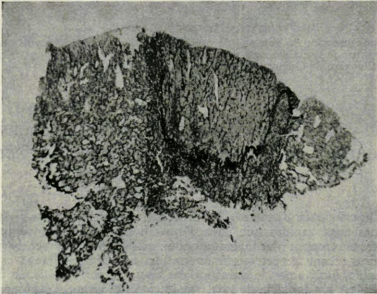
Fig. 11. — Homogreffe Suberites
