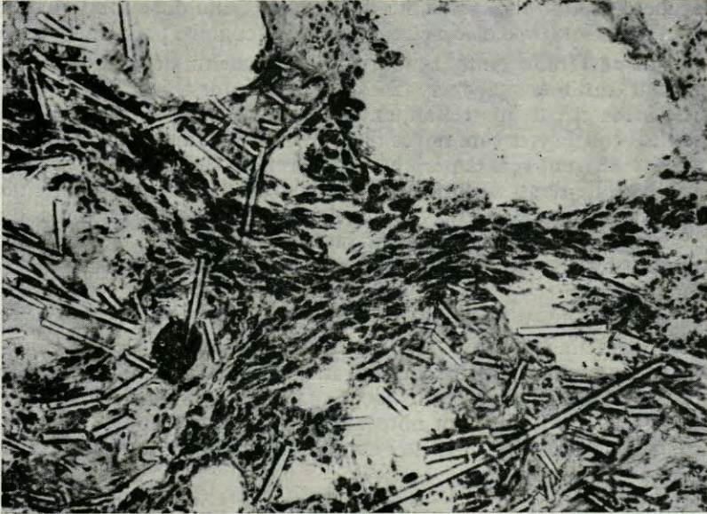
Fig. 10. — Homogreffe Suberites
