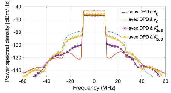
Figure 3. Spectre en bande de base reçu par l'UE avec un canal sans multitrajét (LOS : line-of-sight).
