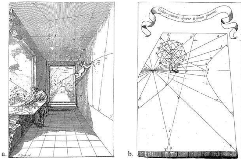
Fig. 1. Immagini del trattato Perspectiva Horaria - sive de horographia gnomonica tum practica tum teoretica ; (a) metodo indiretto: proiezione a partire dal disegno di un quadrante sciatrico orizzontale; (b) proiezione gnomonica e costruzione dell'analemma di Vitruvio (Maignan 1648 da Tolosana, Bibliothèque universitaire de l'Arsenal).
