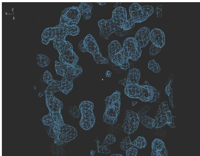
Figure IV_3 : Carte de densité électronique 2F_o - F_c tracée à 1\sigma de la vIPO1 de Z. galactanivorans obtenue après calcul des phases par SHELXE. La solution "main inversée" a été utilisée pour le calcul de la carte.
