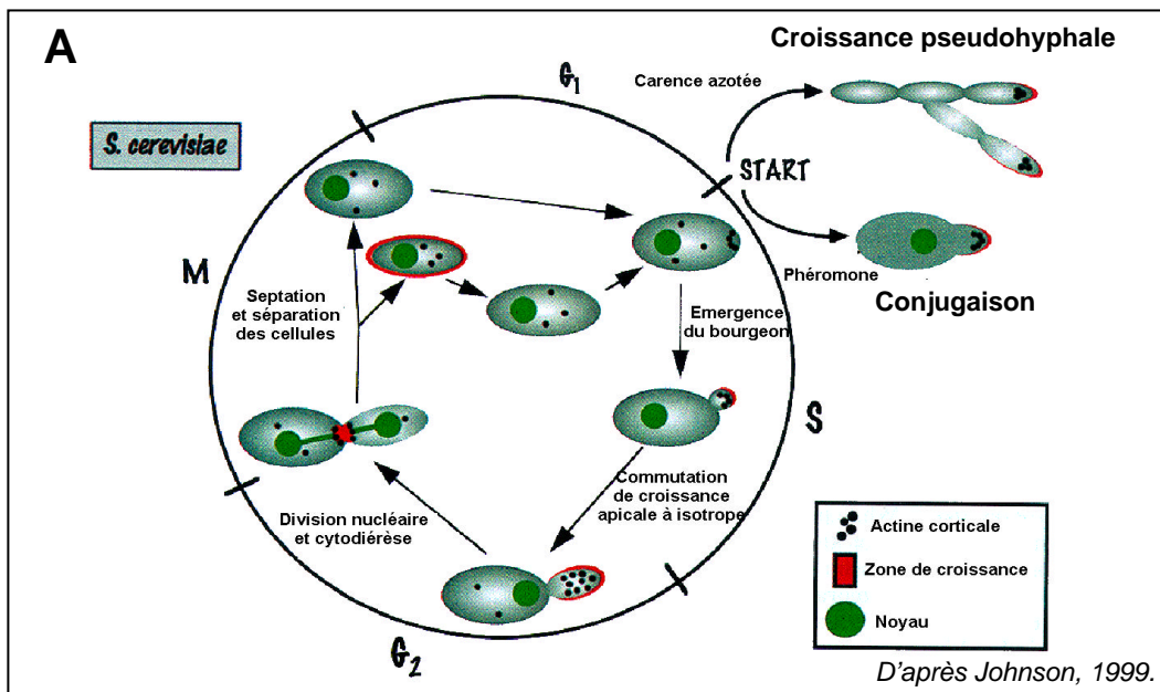
Figure 18 : Cycle cellulaire et morphogénèse chez S. cerevisiae
