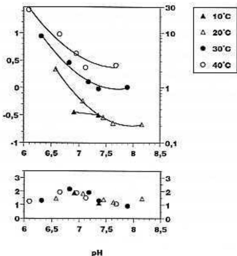
Figure IV.17 : Effets du pH et de la température sur l'affinité ( P_{50} ) et le coefficient de coopérativité ( n_{50} ) de l'hémoglobine vasculaire d' Alvinella pompejana .
