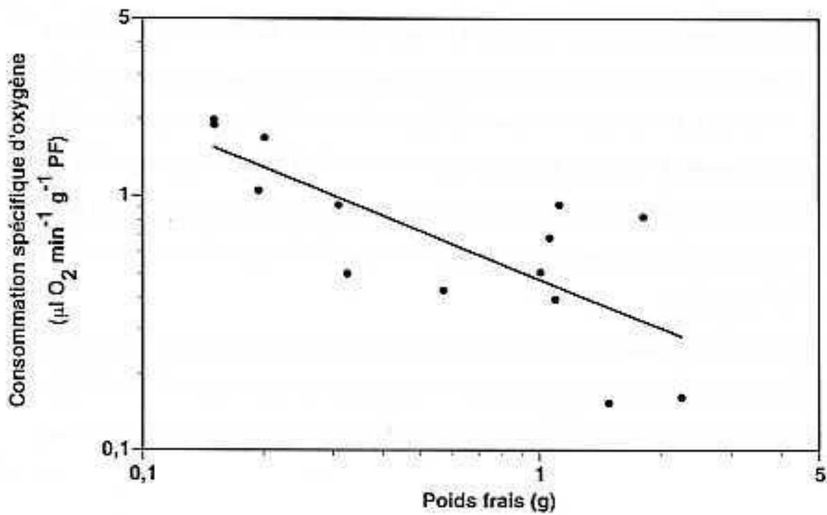
Figure IV.8 : Variation de la consommation spécifique d'oxygène en fonction du poids frais chez Branchipolynoe seepensis .
