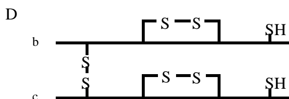
Figure III.26 : Modèle de structure des globines de l'Orbiniidé du Golfe du Mexique avec leurs cystéines. La chaîne d et les linkers ne sont pas représentés car les informations disponibles sur ces chaînes ne sont pas suffisantes pour établir un modèle.
