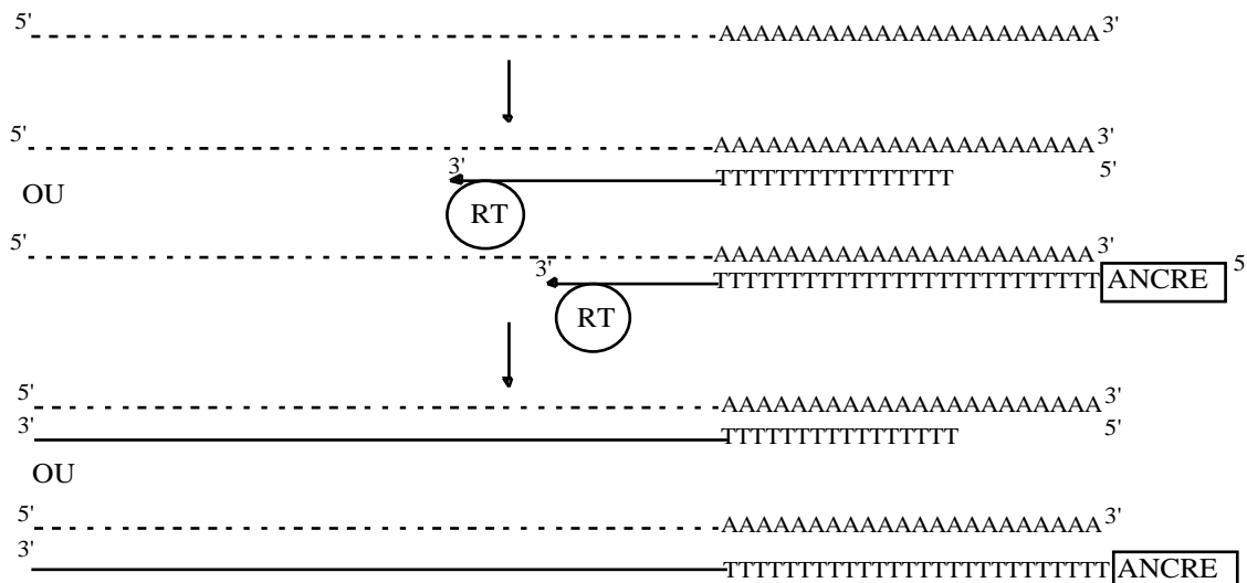
Figure III.9 : Principe de la synthèse des ADN complémentaires par transcription inverse, en utilisant un oligo(dT) ou un oligo(dT) ancré.
