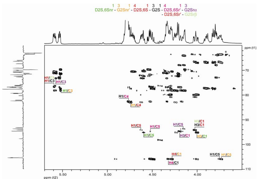
Figure 40 : Spectre hétéronucléaire ^1\text{H}/^{13}\text{C} HMBC à 25 °C du néo- \lambda -carrageaxose.
