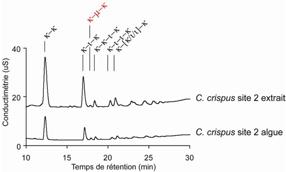
Figure 92 : Comparaison par analyse par HPAEC des produits d'hydrolyse obtenus par action de la \kappa -carragénase sur le carragénane extrait de C. crispus site 2 et directement sur la paroi de l'algue broyée.
