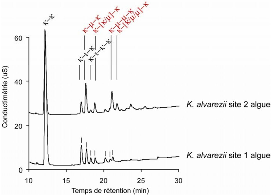
Figure 91 : Comparaison par analyse par HPAEC des produits d'hydrolyse obtenus par action de la \kappa -carragénase directement sur la paroi des algues K. alvarezii des sites 1/2.
