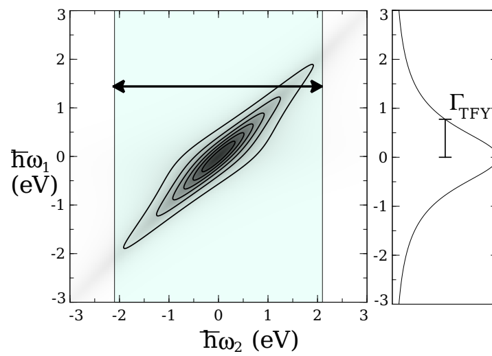
FIG. 1.12 – Largeur pour le rendement en fluorescence total (TFY). A gauche, courbes de niveau de la fonction f(\hbar\omega_1, \hbar\omega_2) . A droite, valeur de l'intégrale \int f(\hbar\omega_1, \hbar\omega_2)d(\hbar\omega_2) . La largeur de la courbe obtenue, qui est celle du TFY, est celle du niveau 1s.
