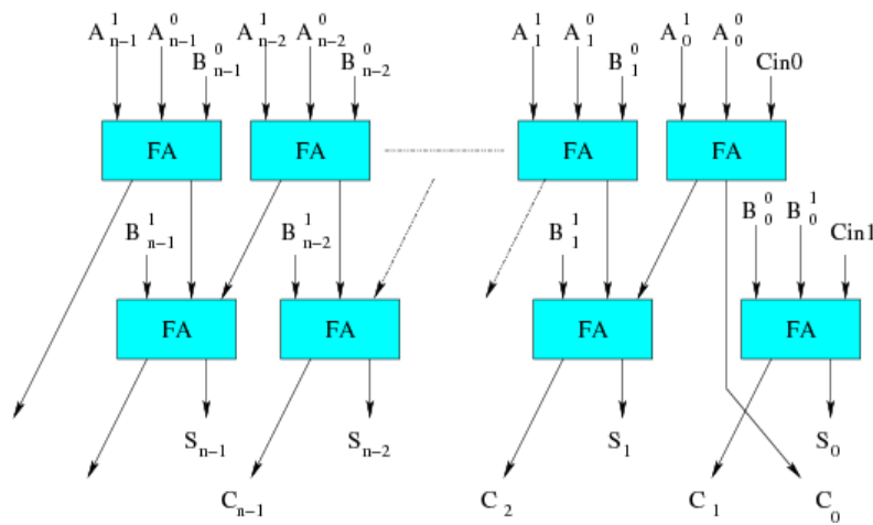
FIG. 2.3 – Additionneur redondant
