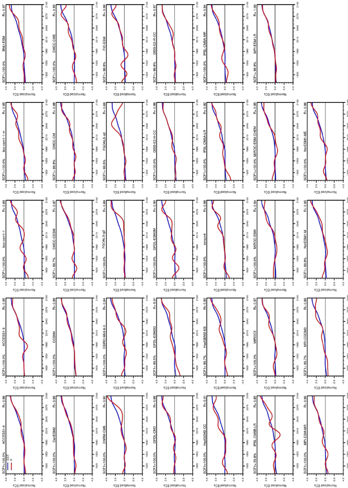
FIGURE 6.8 – Première Composante principale (CP) issue de la SVD long terme des précipitations (courbe bleue) et des SST (courbe rouge) en été 1901-2099. La SVD a été calculée avec les champs de précipitations sur le SAHEL (18°W-10°E ; 10°N-20°N) et les anomalies de SST globales.
