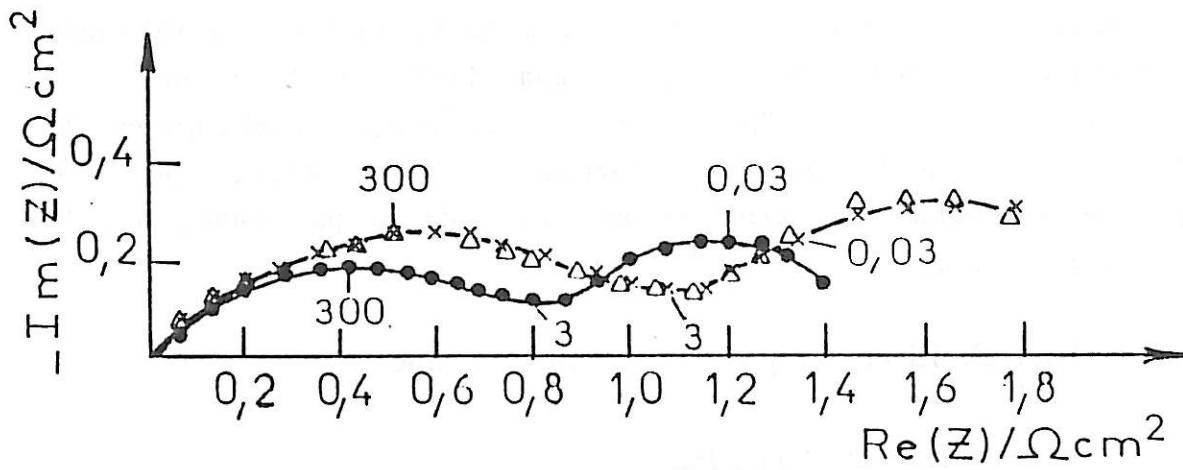
Figure II.3.7 : Evolution de l'impédance de la poudre de zinc au cours du temps
