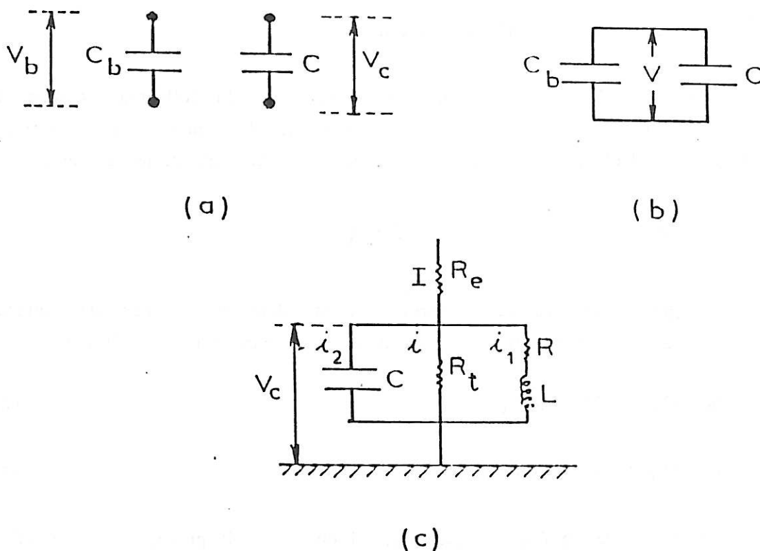
Figure III.4.1 : Schéma électrique caractérisant le collecteur de zinc avant (a), pendant (b) et après (c) le choc bille-collecteur.
